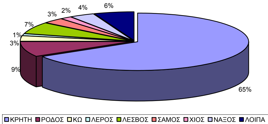
Συνολική παραγωγή 85 Αιολικών Πάρκων 54.355,89 MWh
