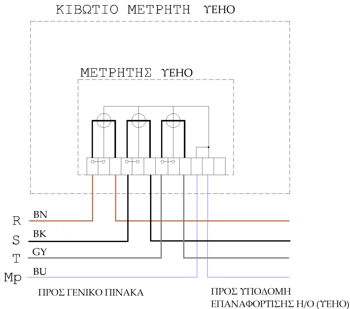
Σχήμα 1: Μονογραμμικό Διάγραμμα Μετρητικής Διάταξης τριφασικού μετρητή ισχύος έως 55 kVA
