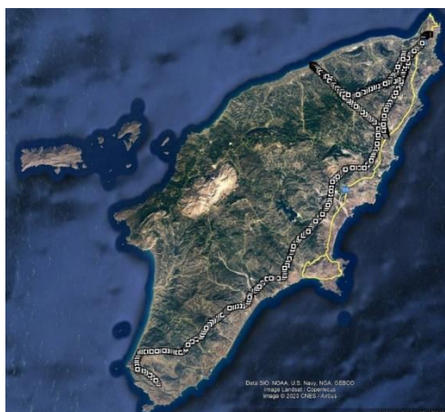
Εικόνα 1: Ζώνη δουλείας των γραμμών μεταφοράς ηλεκτρικής ενέργειας (150kV) στο νησί της Ρόδου.
