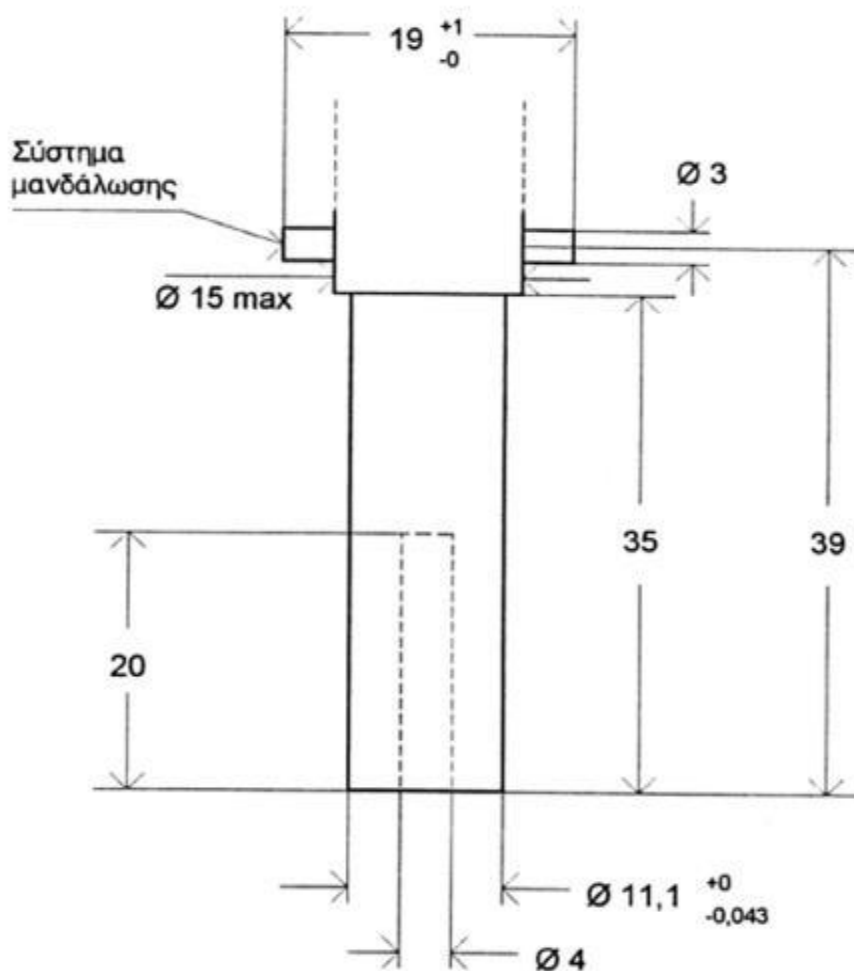
Σχέδιο 1: Βύσμα ειδικού ρευματοδότη
